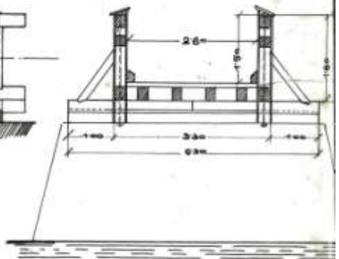
QUERSCHNITT AB
